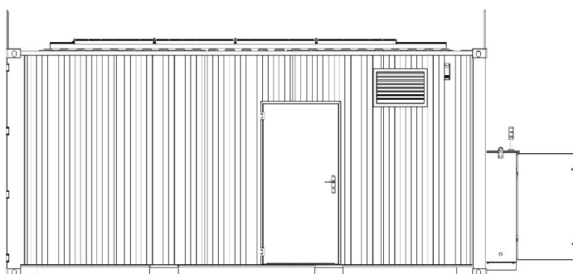
Rysunek 2: Widok poglądowy kontenera (strona prawa). Zaznaczenie miejsca wykonania otworów technologicznych pod czerpnię powietrza oraz drzwi.
