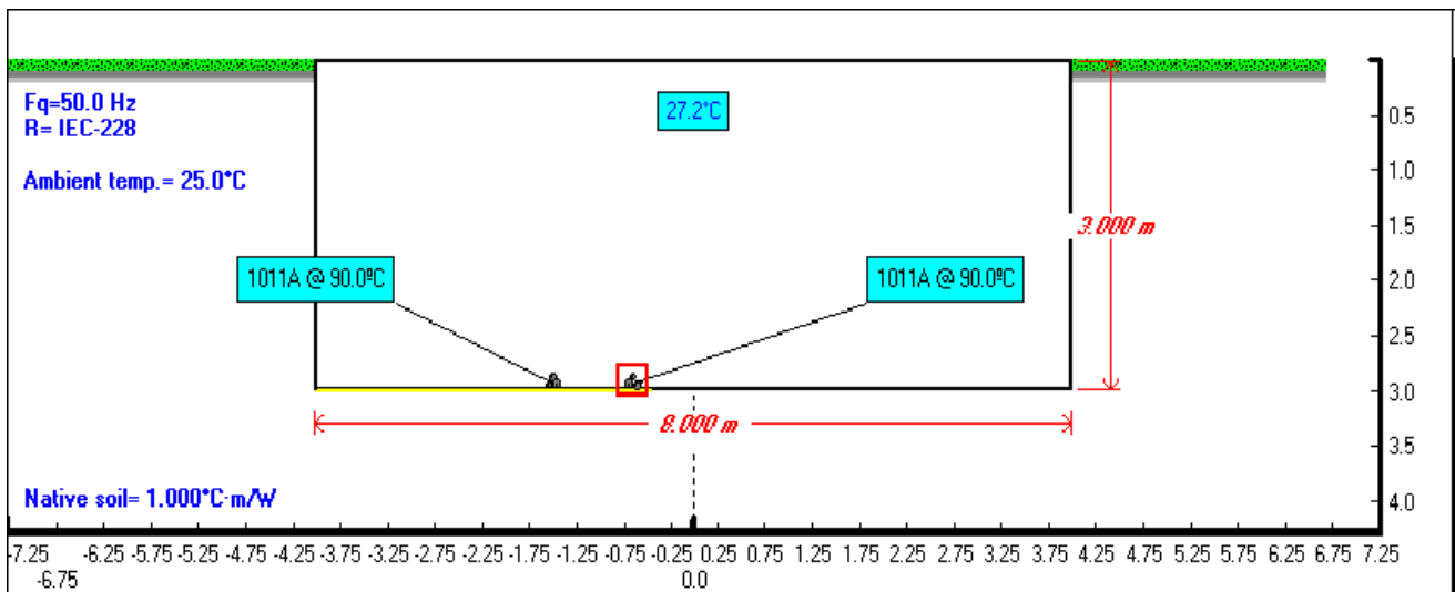
Abbildung 3. Dreieckanordnung, zwei Systeme auf dem Boden. Lastfaktor 1.0.
