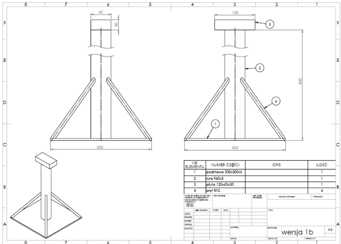
Rysunek nr 2 - Stojak typ 2
