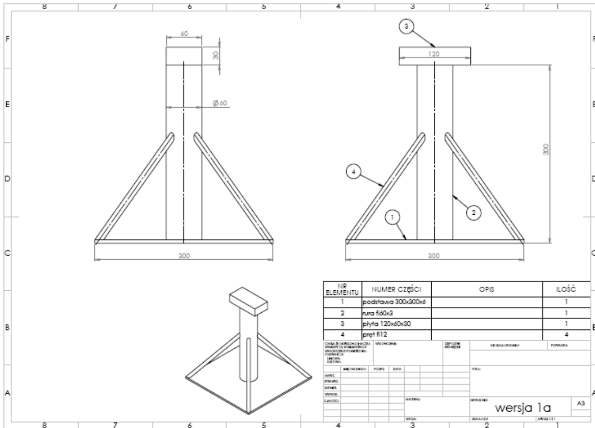
Rysunek nr 1 - Stojak typ 1
