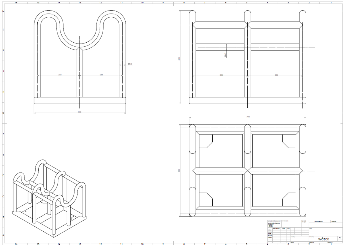
Rysunek nr 5 – wózek transportowy
